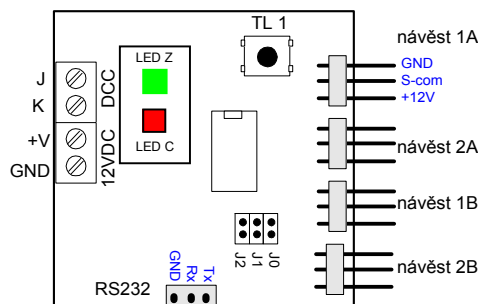
ND4 V2.0 opravené pozice LED
