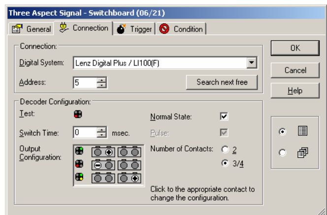
B) ovládání 3 znakového návěstidla 1B, DCCadr=1
