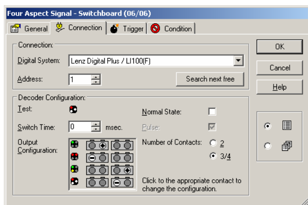
Obr. A) ovládání 4 rychlostního návěstidla
